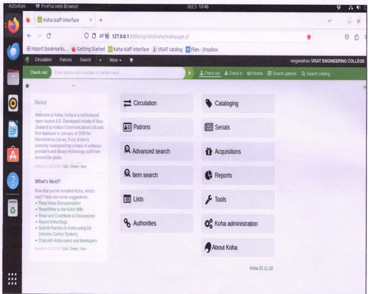
ILMS Software-KOHA
