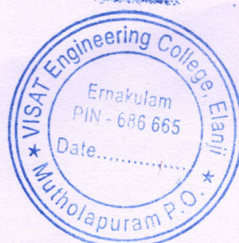
ILMS Software-KOHA
